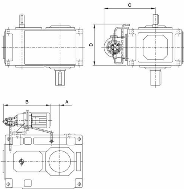
H3.V, H4.V
