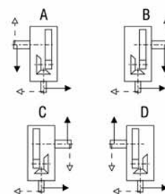
布置形式 Design:
