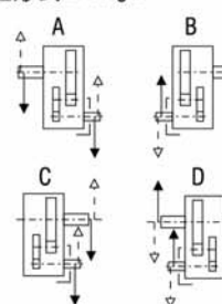
布置形式 Design:
