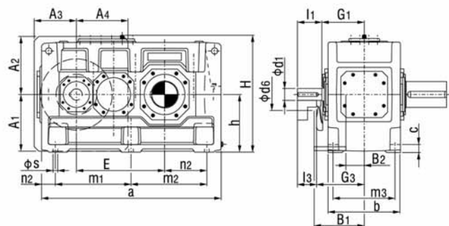
H2SH、H2HH、H2DH
