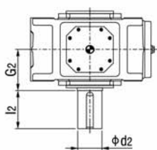
B4SV 实心轴 Solid shaft
