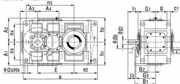
H2HM、H2DM
